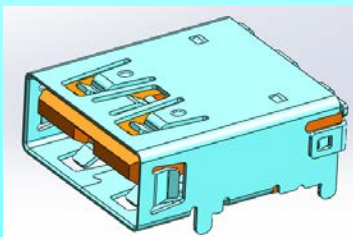
QCA母座 R/A 90度
