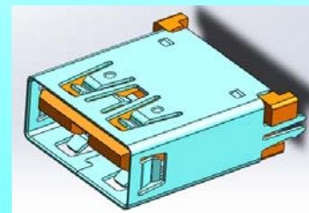
QCA母座 DIP 180度
